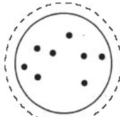
SAGITTARIUS, the Archer
